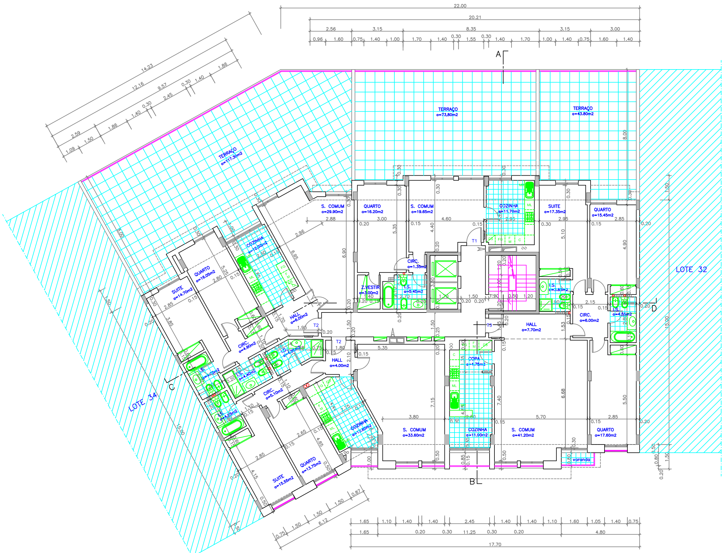
PLANTA DO R/CHÃO
