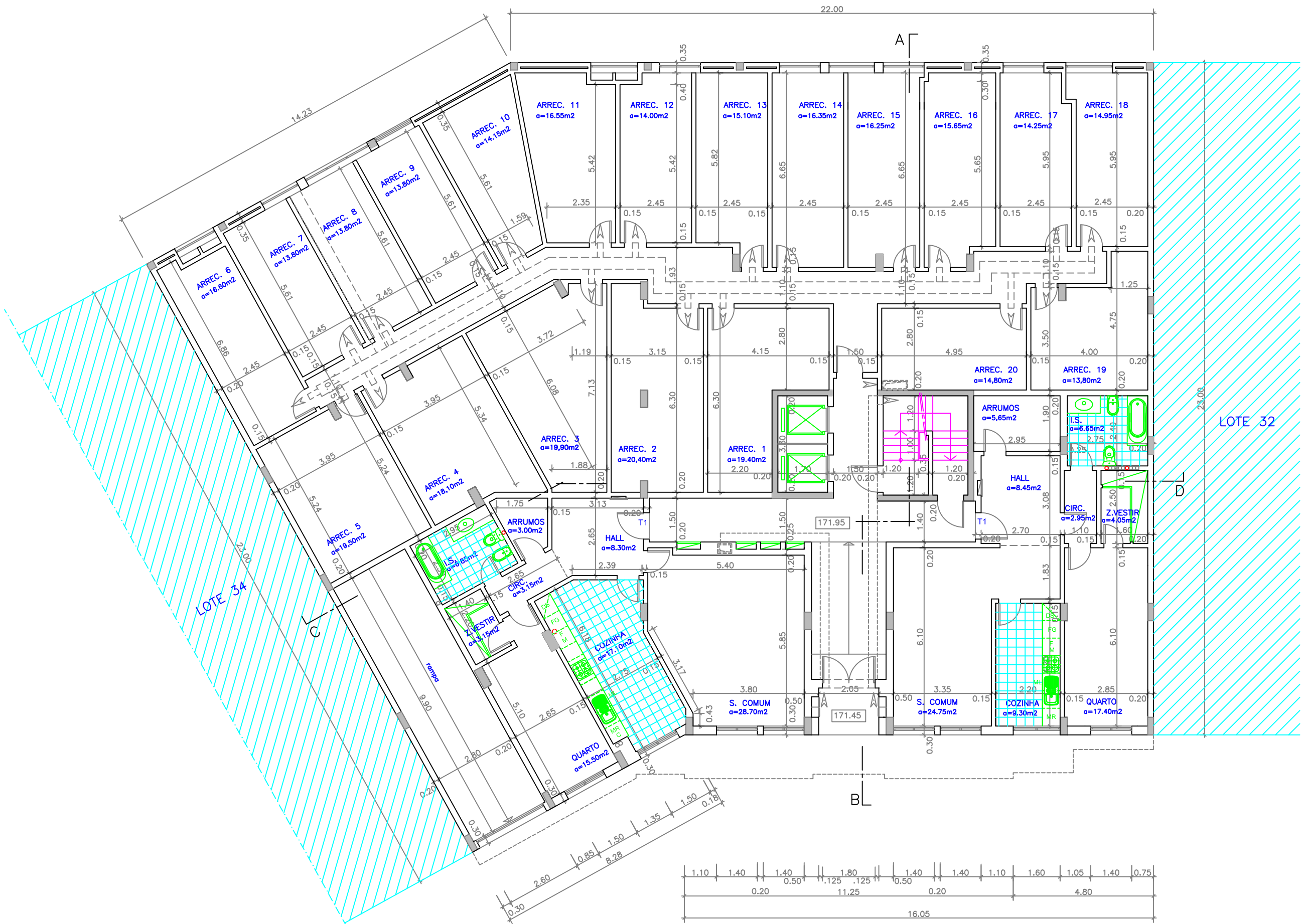
PLANTA DA CAVE
