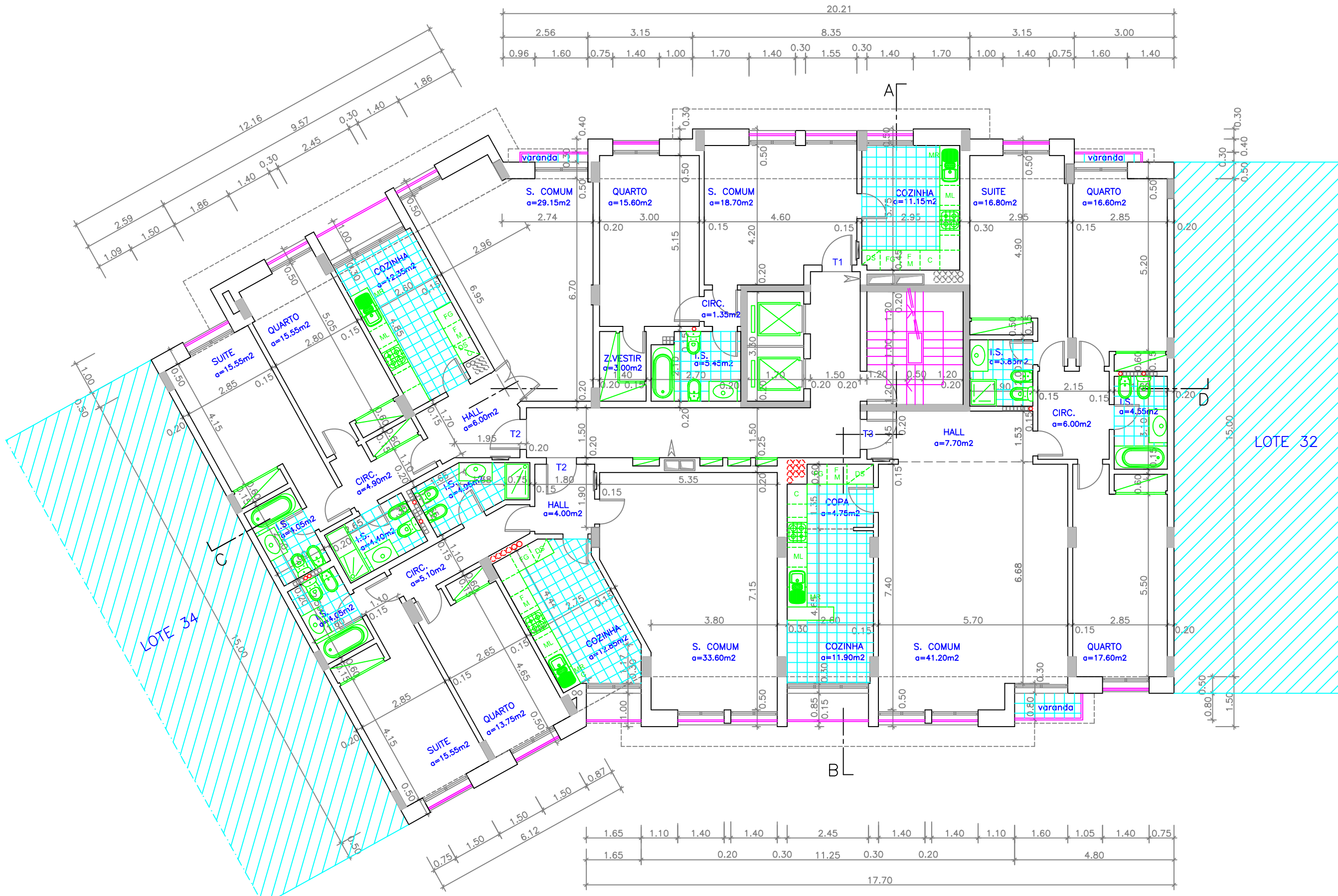
PLANTA DO 1º AO 4º ANDAR
